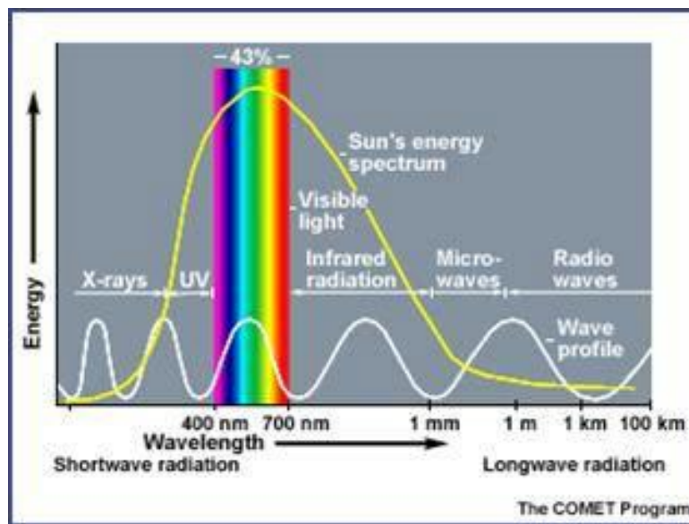
Fig: The solar spectrum.
