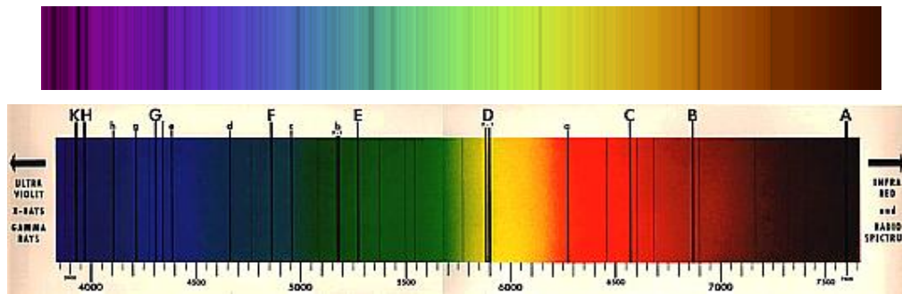
Fig : The Solar Spectrum
