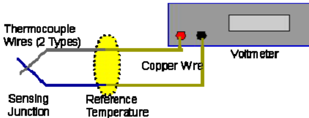
Fig: Thermocouple
