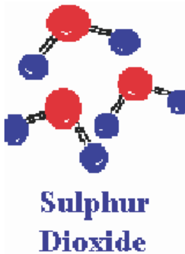
Fig: Acid Rain
