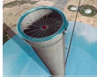
Solar Chimney(SBP)
